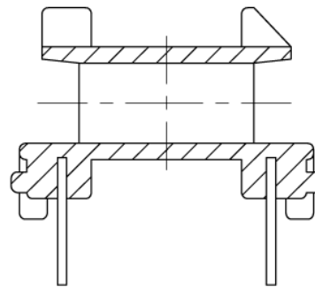
SEC. A-A
