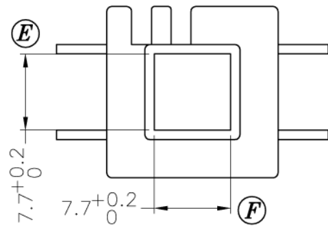
SEC.A-A
