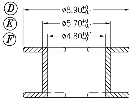
SEC A-A
