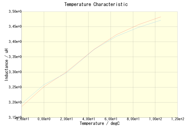
CLF10040T-3R3N(DC = 0A)
