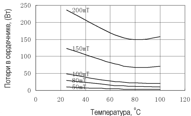
Потери на частоте 100 кГц
