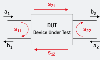
Figure 2: S parameters
