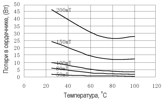
Потери на частоте 50 кГц
