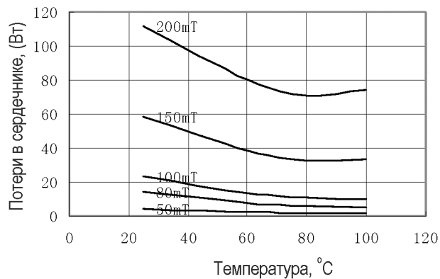
Потери на частоте 100 кГц
